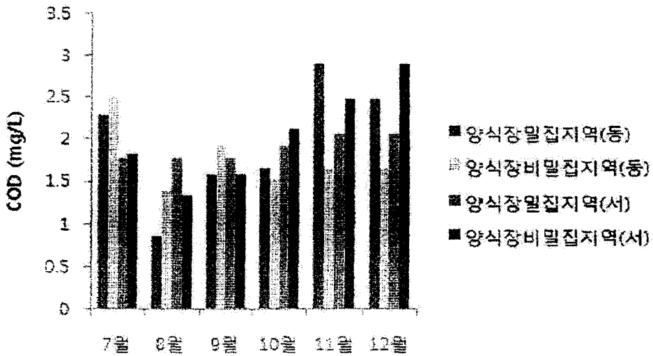
그림 3-17. 화학적산소요구량(COD) 분석결과
