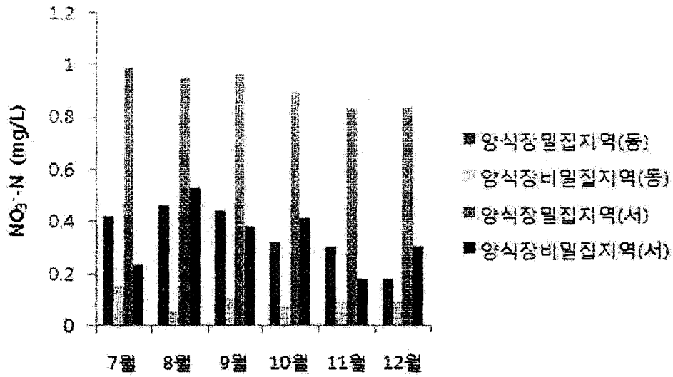
그림 3-12 질산질소 분석결과
