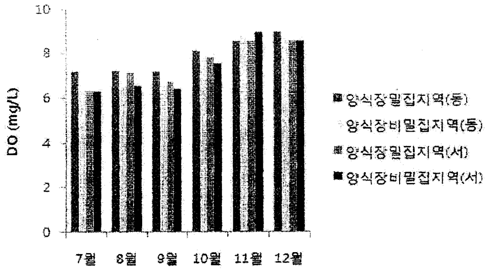
그림 3-18. 용존산소(DO) 분석결과
