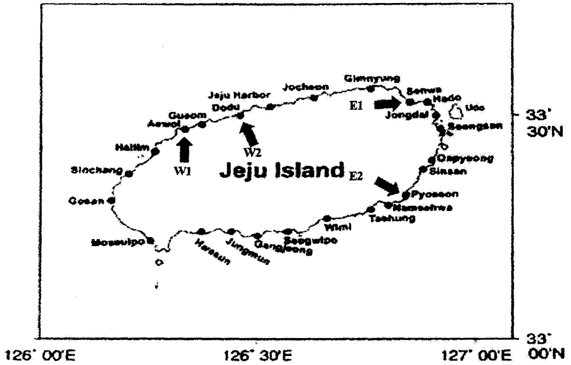
그림 3-2 수생환경 모니터링 조사지점
