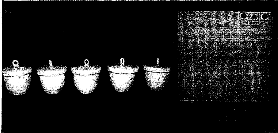
그림 3-1. 분석에 사용된 기자재
