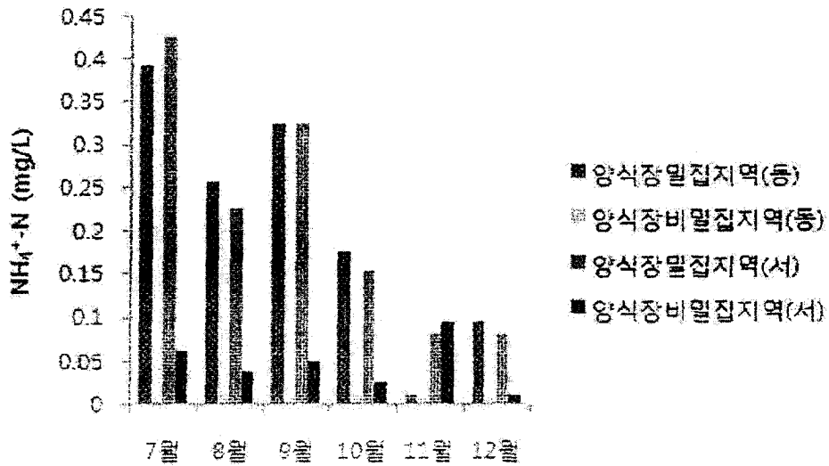
그림 3-13. 암모니아질소 분석결과
