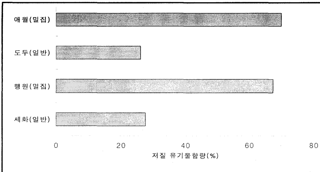
그림 3-11. 저질 유기물 함량 측정결과
