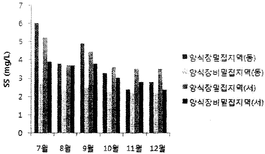
그림 3-16. 부유물질(SS) 분석결과
