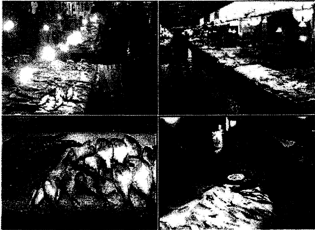
그림 3-8. 어류 채집 과정
