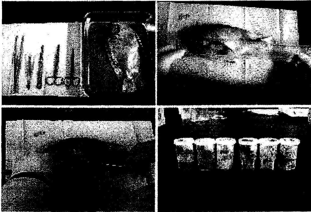
그림 3-7. 위 내용물 채취과정
