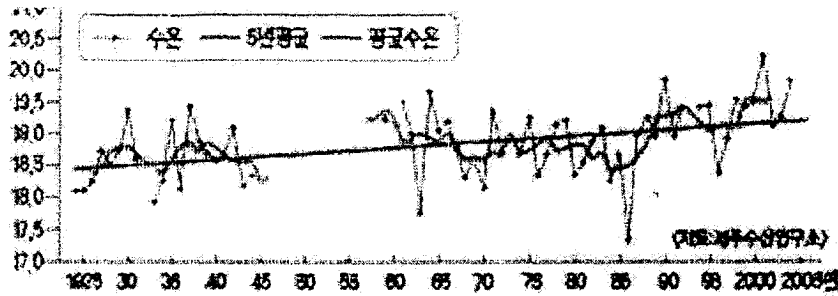
그림 1-2 마라도 연안의 연평균 수온상승추세
