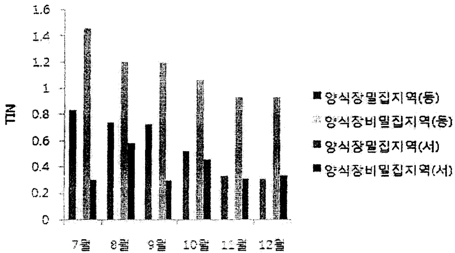
그림 3-15. 총 무기질소(TIN) 분석결과
