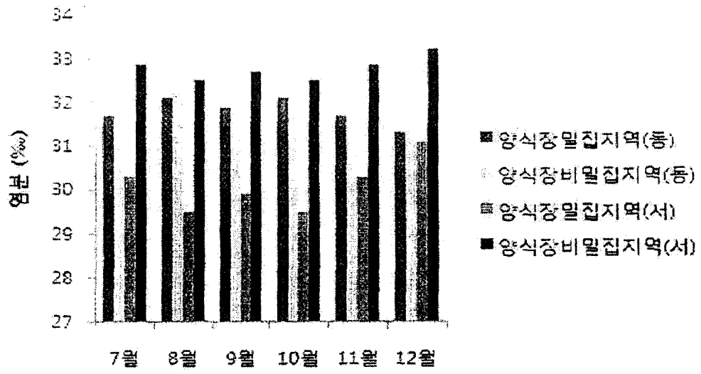
그림 3-20. 임분 분석결과
