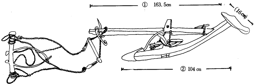
〈그림 13〉 쟁 기
