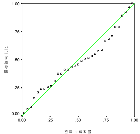
그림 6 표준화잔차의 분포
