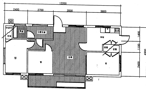
그림13. 후생주택의 평면(18평)
